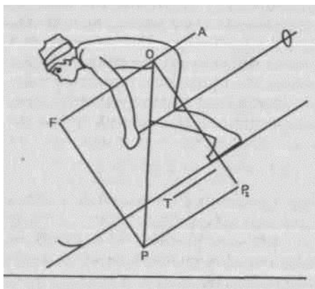
Рис. 1. Силы, действующие на лыжника на склоне
