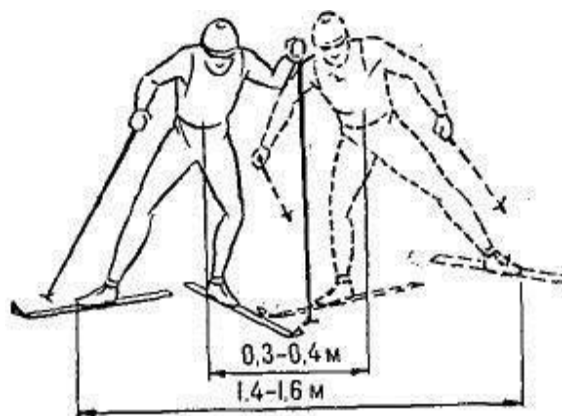
Поперечные колебания в коньковом одновременном двухшажном ходе
