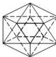
икосаэдр
