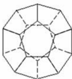
додекаэдр
