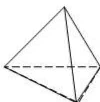
тетраэдр
