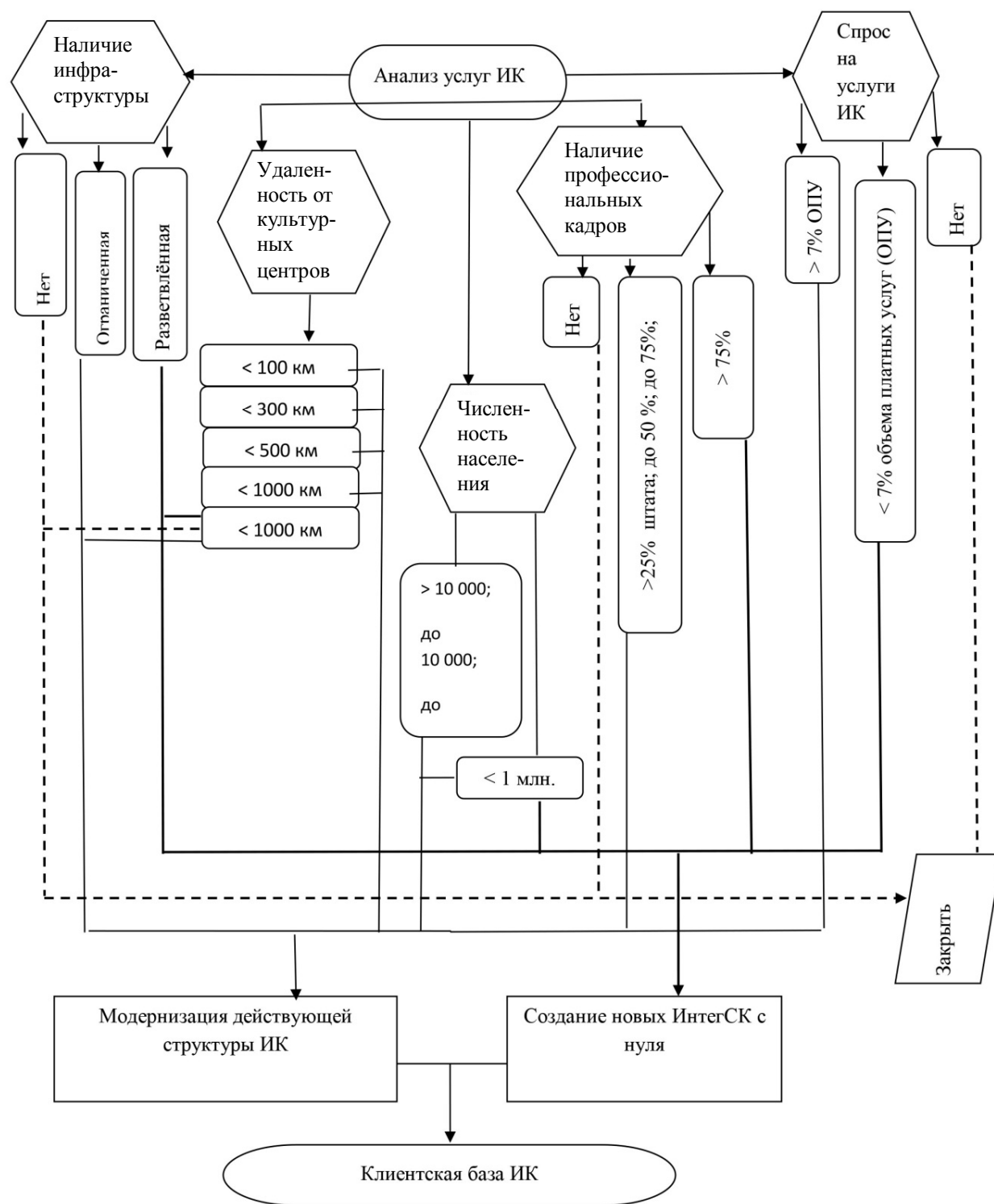
Рисунок 1. Алгоритм формирования информационно-аналитической базы данных индустрии культуры
