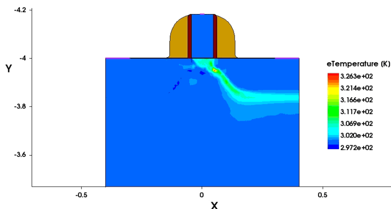
Моделирование распределения температуры в pМОП-транзисторе
