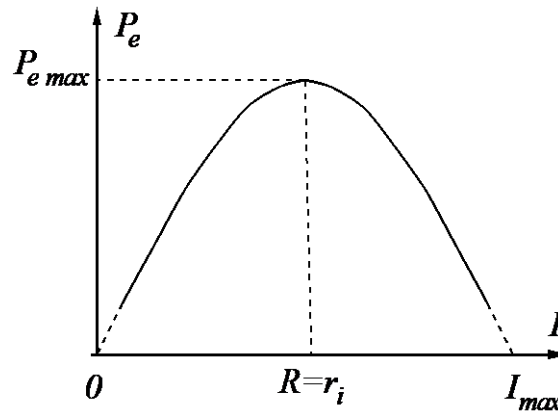
Рисунок 9.2. График зависимости полезной мощности от силы тока
