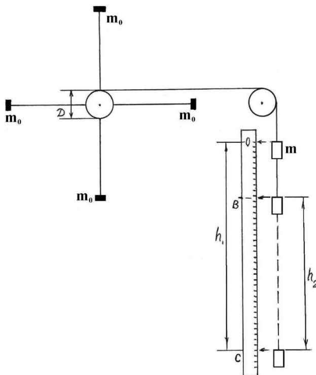
Рисунок 2.7. Схема опытной установки
