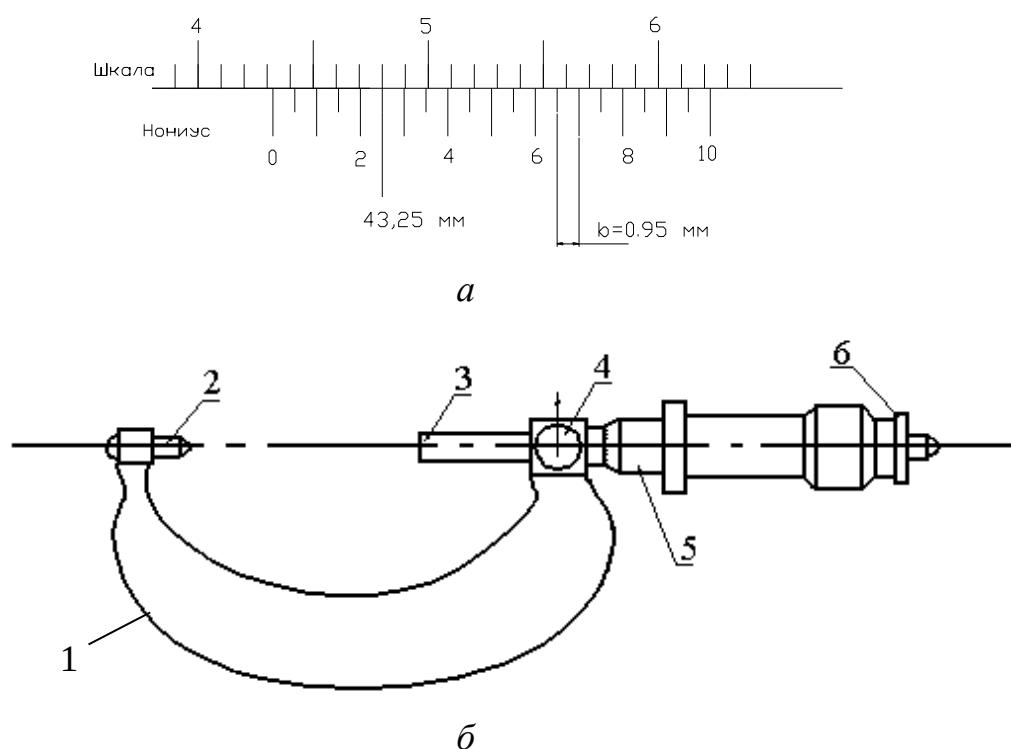
Рисунок 1.1. а – нониус штангенциркуля; б – гладкий микрометр МК: 1 – скоба, 2 – пятка, 3 – микрометрический винт, 4 – стопор, 5 – барабан, 6 – трещотка
