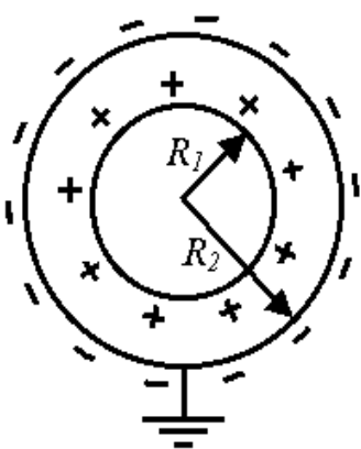
Рисунок 8.1. Сферический конденсатор
