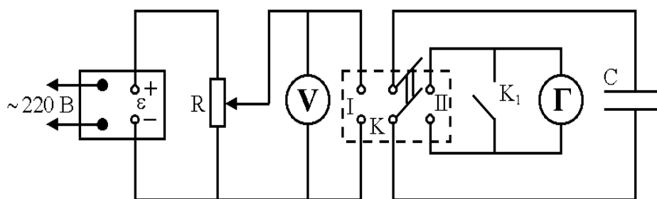
Рисунок 8.3. Электрическая схема установки:
