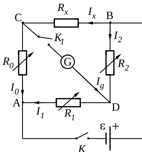
Рисунок 10.3. Мост Уитстона
